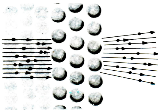
Partículas \alpha assim “atravessariam” o ouro (Thomson).
